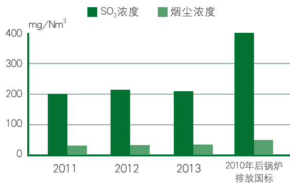
4# 烟囱2011-2013年SO 2 烟尘浓度
